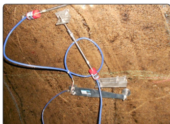
♦ Installation typique de fissuromètres 3D et géophone en tunnel
